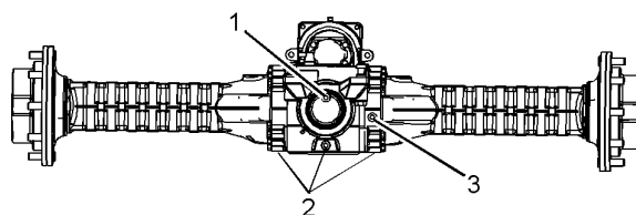
Рисунок 2 g03590601 (1) Сливная пробка заднего дифференциала (2) Заглушка отверстия для проверки уровня масла заднего дифференциала (3) Сливная пробка заднего дифференциала
